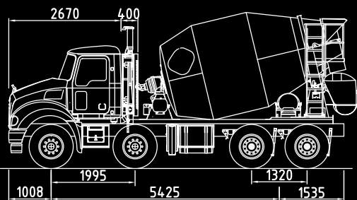
METRO-LINER 8X4 AGITATOR
