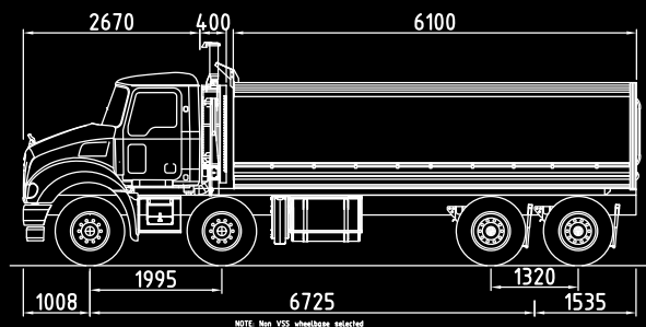
METRO-LINER 8X4 RIGID TIPPER
