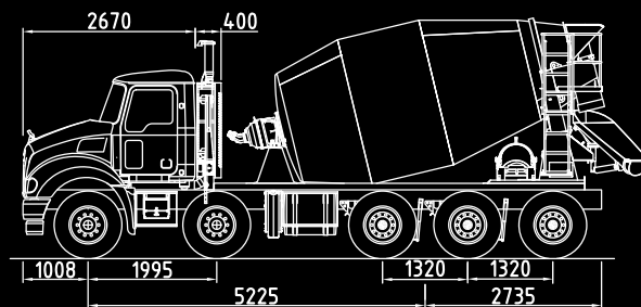
METRO-LINER 10X4 AGITATOR
